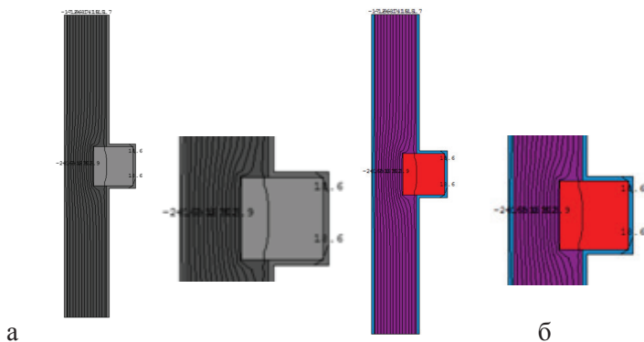
Рис. 2. Распределение плотности теплового потока по сечению наружной стены, выполненной кладкой из ячеистобетонных блоков, и колонны: а – ча-
