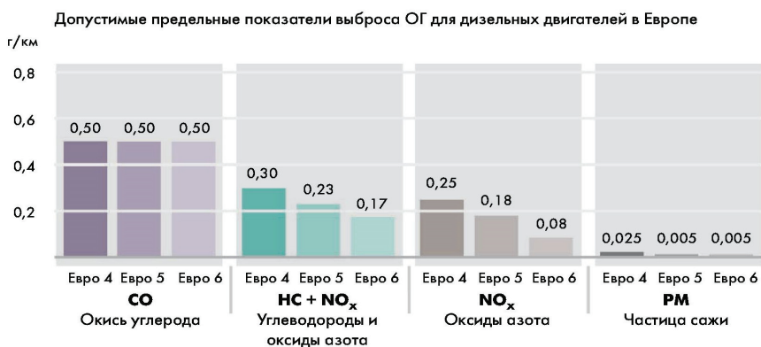
Рис. 1. Допустимые предельные показатели выбросов ОГ для дизельных двигателей в Европе
