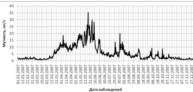
Рис. 3. – Ряд наблюдений за 2007 год по показателю мутность
