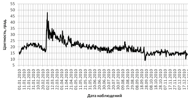
Рис. 4. – Ряд наблюдений за 2010 год по показателю цветность
