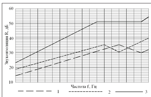
Рис. 1. Частотная характеристика звукоизоляции двойного ограждения разной толщины
