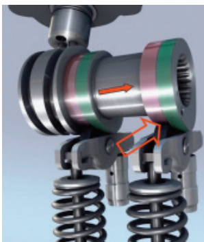
Рис. 2. 1 из 2 цилиндров отключен
