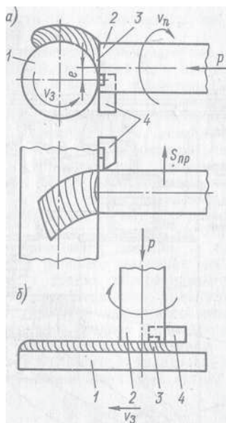
Рис. 1. Схема наплавки вращающимся прутком на цилиндрическую (а) и плоскую (б) поверхность
