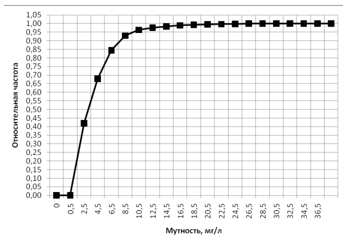
Рис. 1. – Интегральная функции распределения показателя мутность
