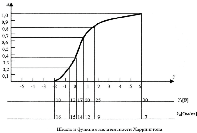
Рис. 1. Шкала и функции желательности Харрингтона
