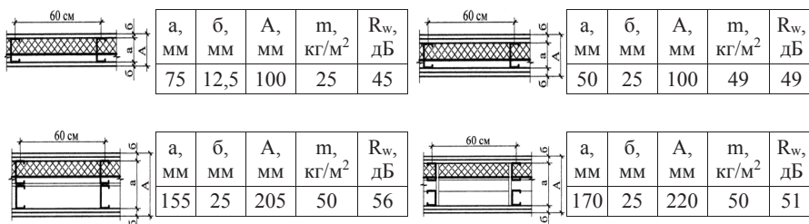
Рис. 2. Технические и акустические характеристики двойных перегородок из гипсокартонных листов на стальном каркасе
